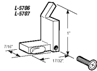
ACORN SWIVEL
